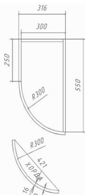
ШКАФ 316-550
