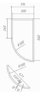
ШКАФ 316-560
