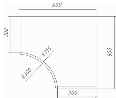
ШКАФ 600-600-300
