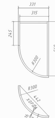
ШКАФ 331-560
