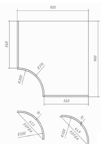
ШКАФ 900-900-560
